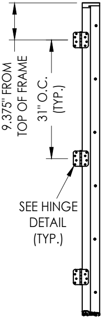
HINGE JAMB
